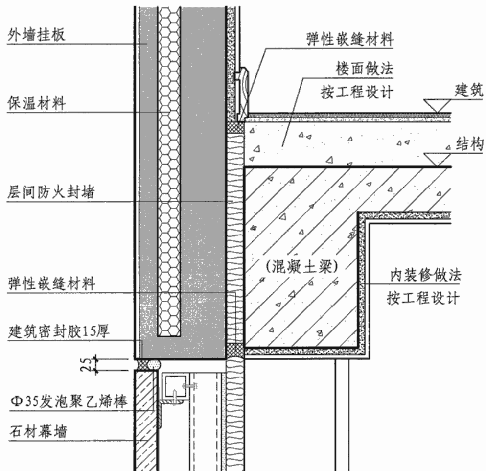
① 墙板底部与幕墙交接构造
