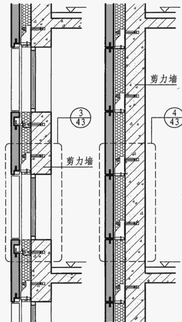
A-A
