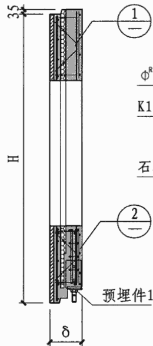
1-1
