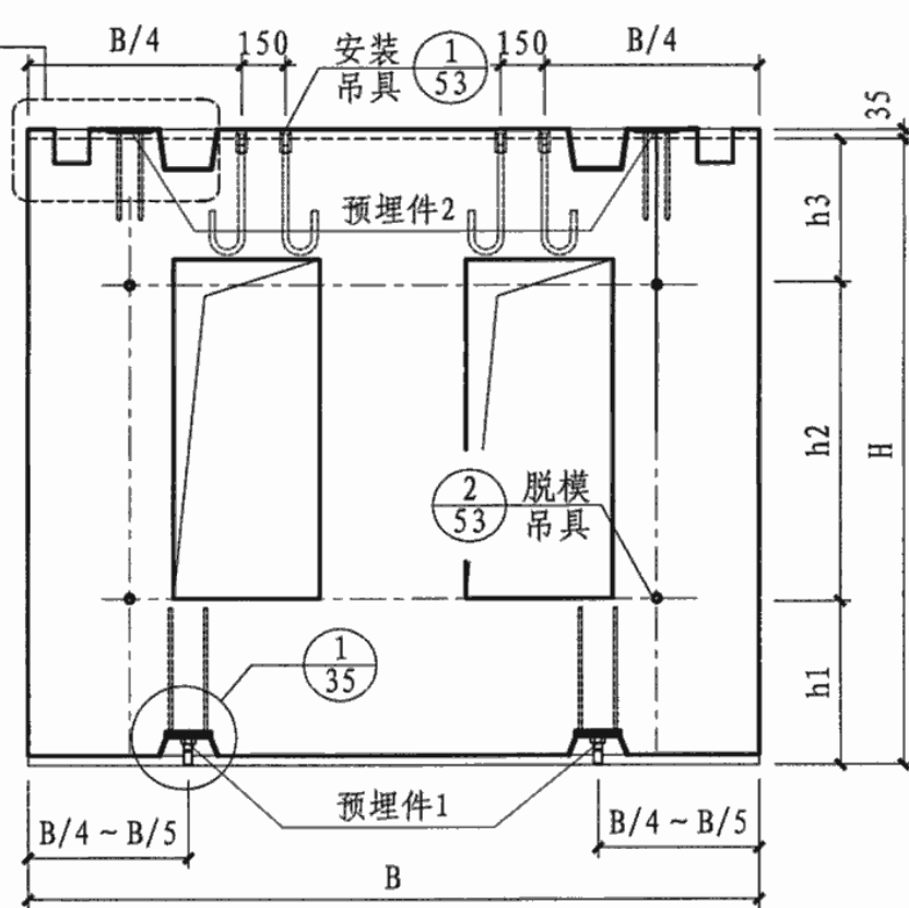
挂板背立面
