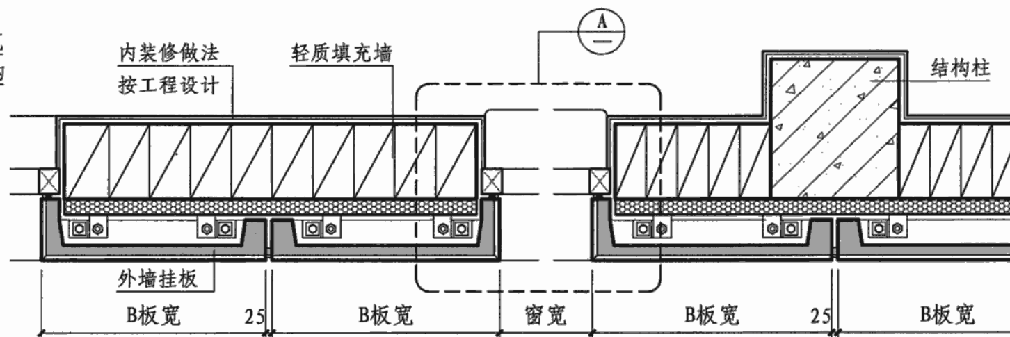
② 装饰板墙身横剖面
