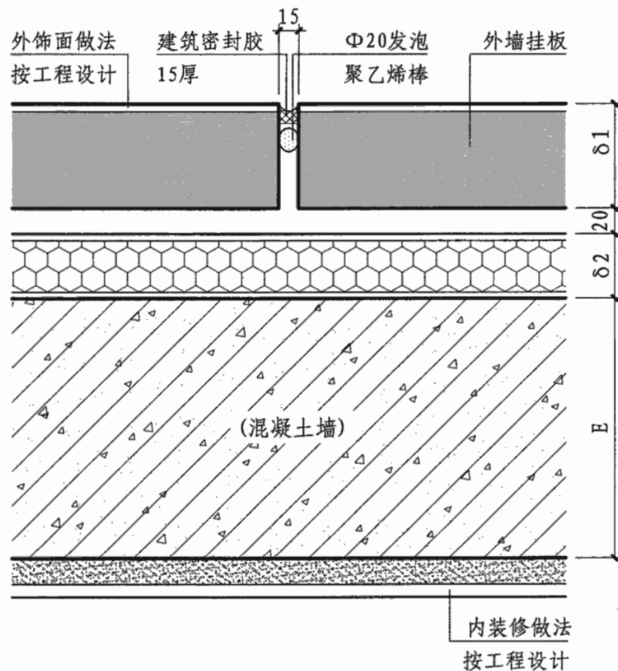
② 外墙挂板垂直缝横剖面构造
