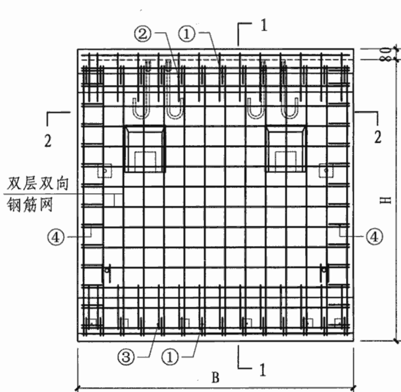
挂板背立面
