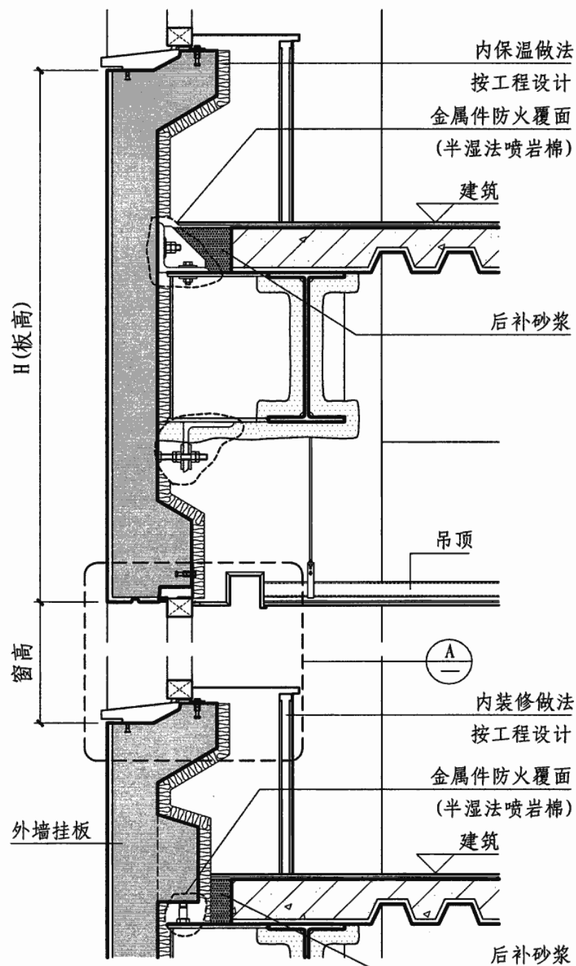
1 横条板墙身剖面
