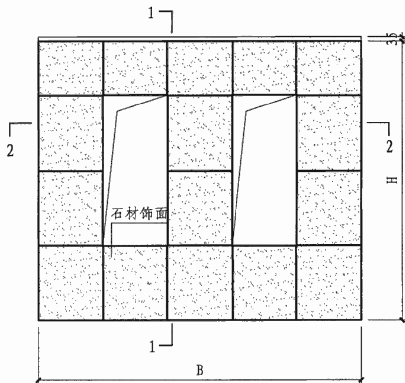
挂板正立面
