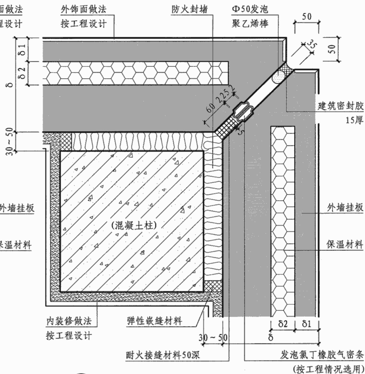
② 外墙挂板阳角横剖面构造
