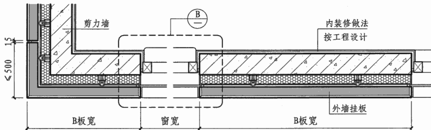
② 装饰板墙身横剖面
