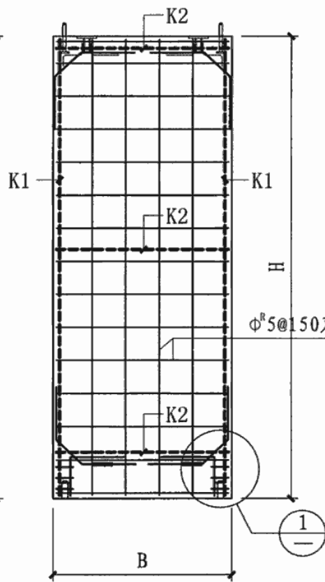
挂板配筋示意
