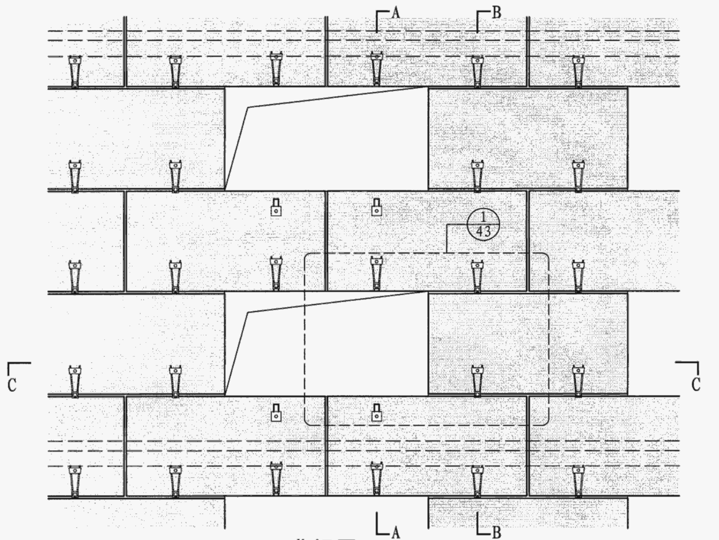
背视图
