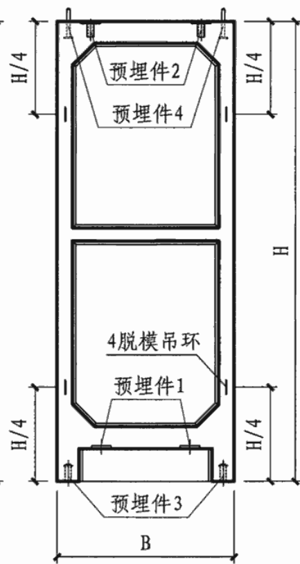
挂板背立面
