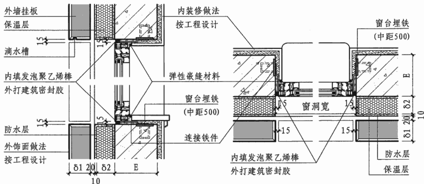
③ 窗洞口纵剖面构造
