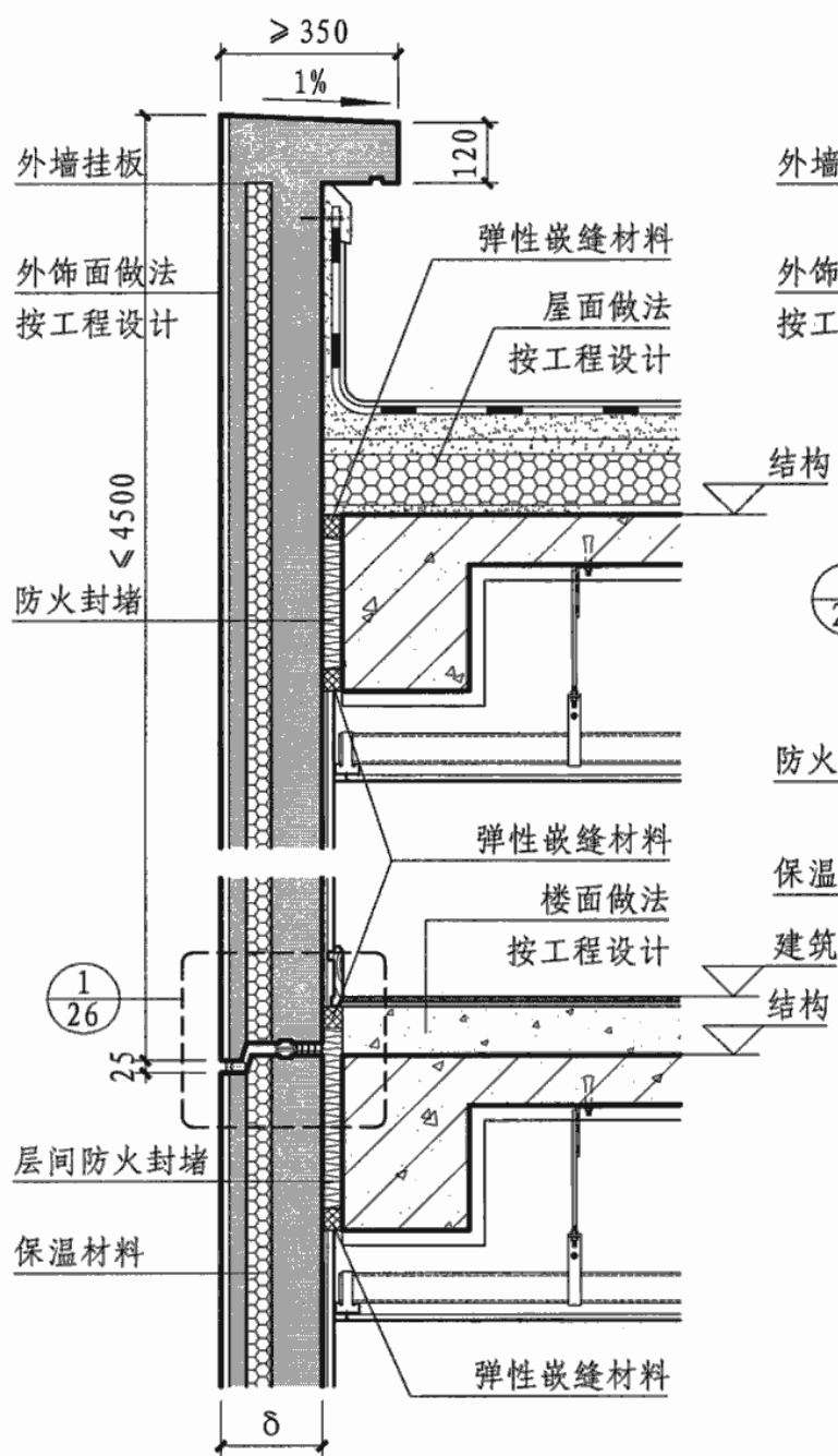
① 女儿墙墙身剖面详图
