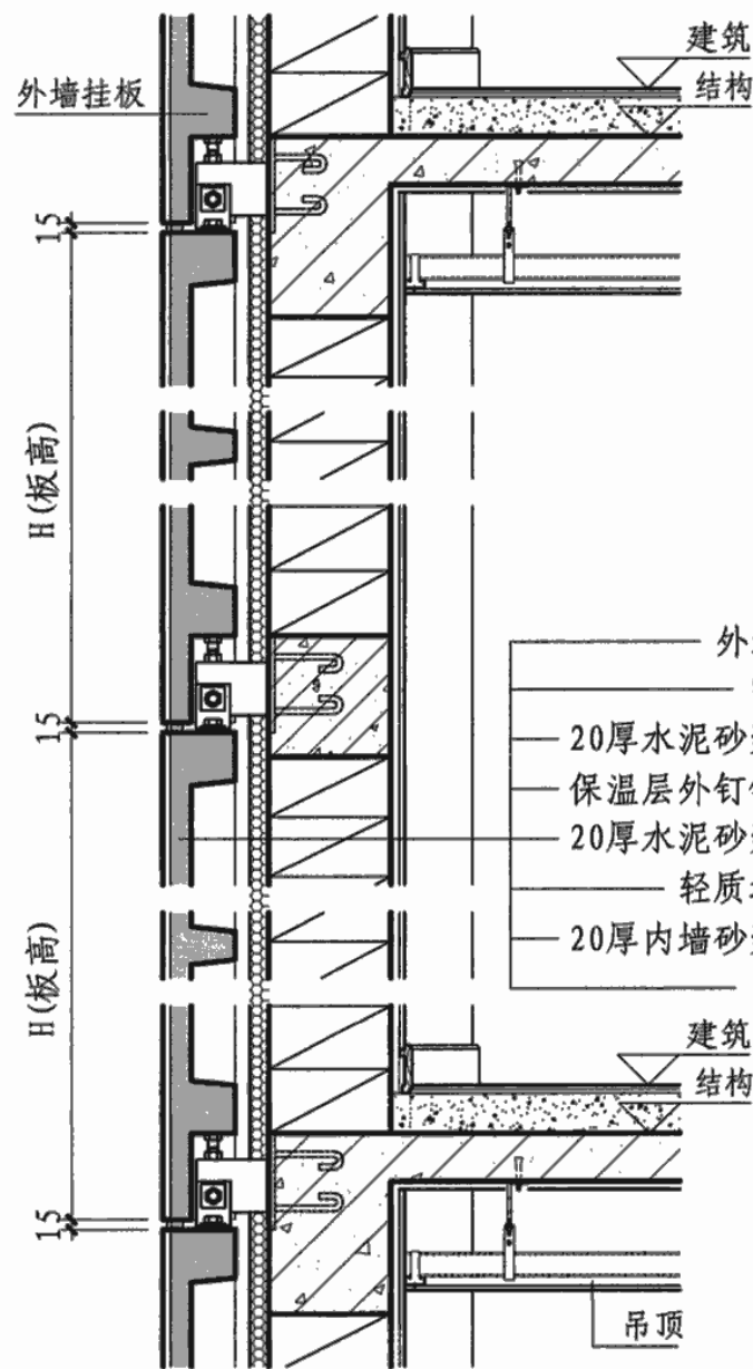
① 装饰板墙身纵剖面
