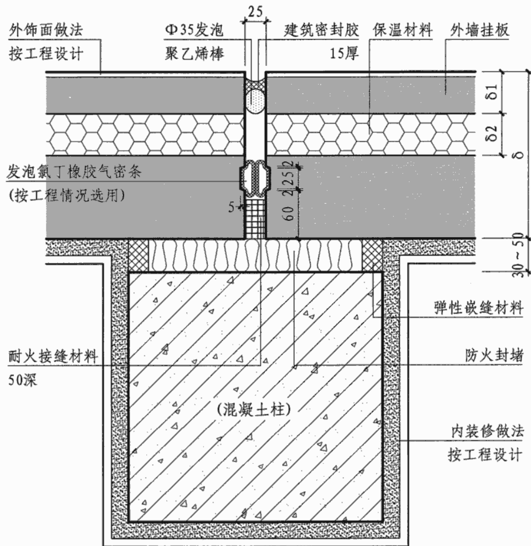
② 外墙挂板垂直缝横剖面构造
