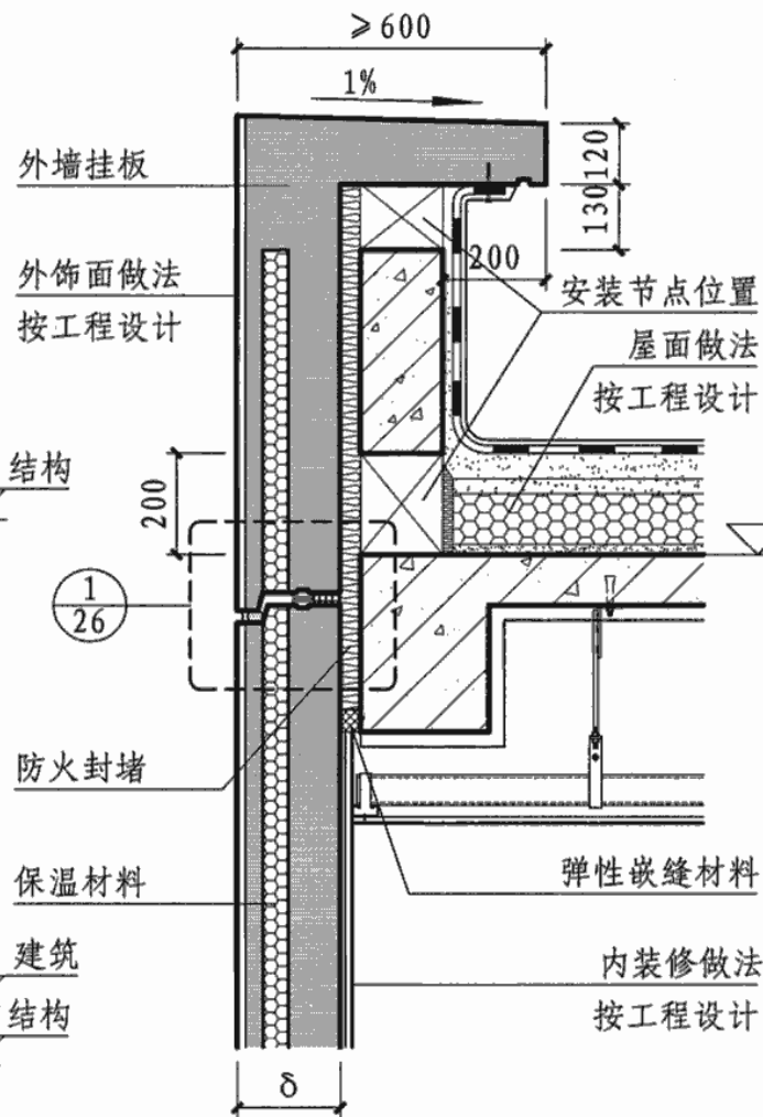
② 女儿墙墙身剖面详图
