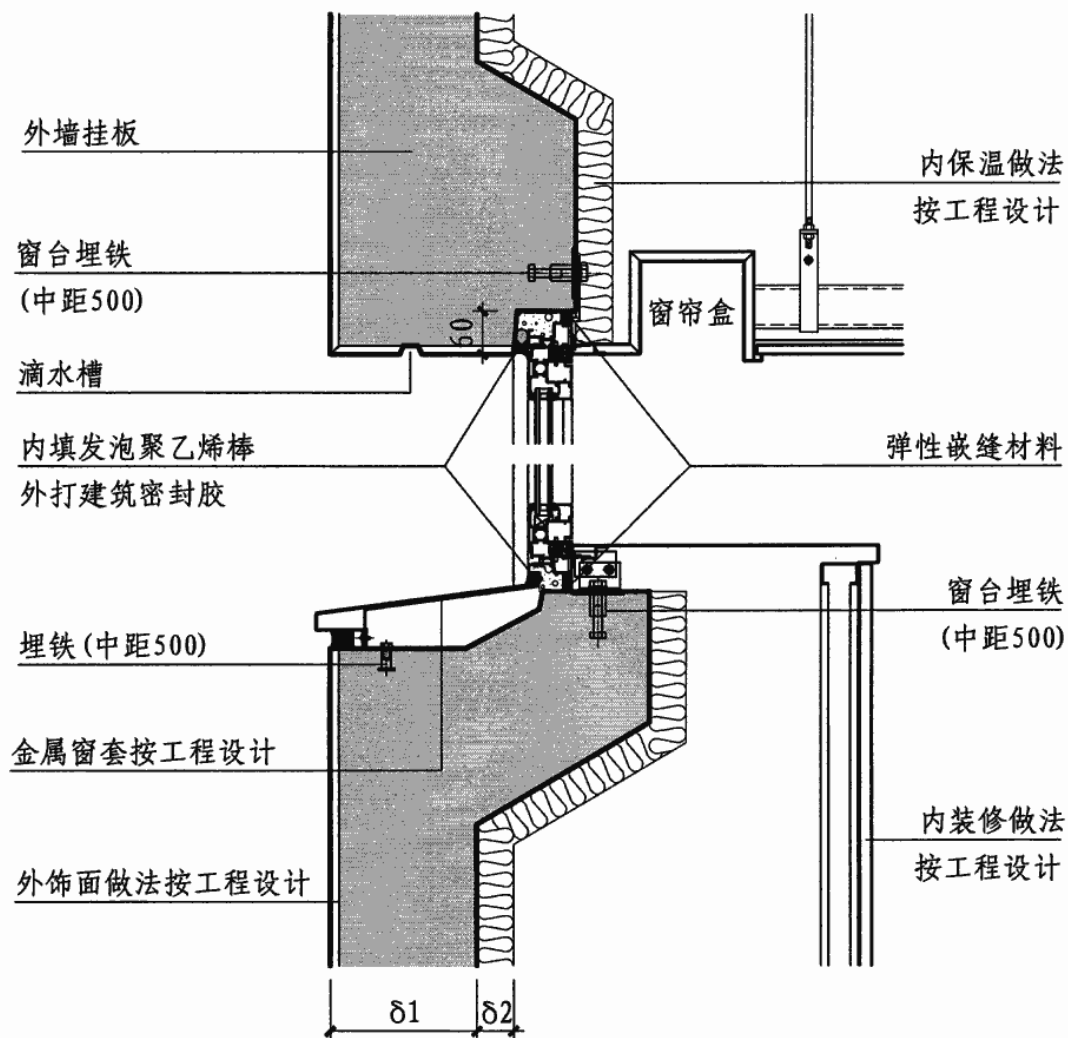
A 窗洞口纵剖面构造
