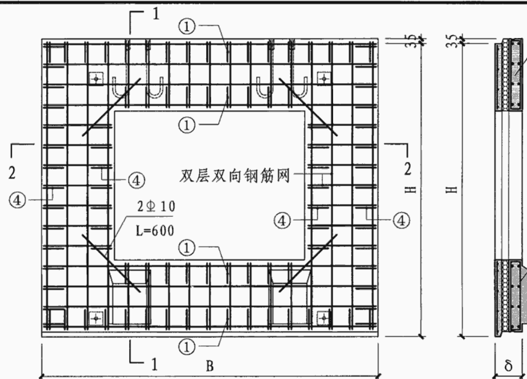
挂板结构层配筋示意
