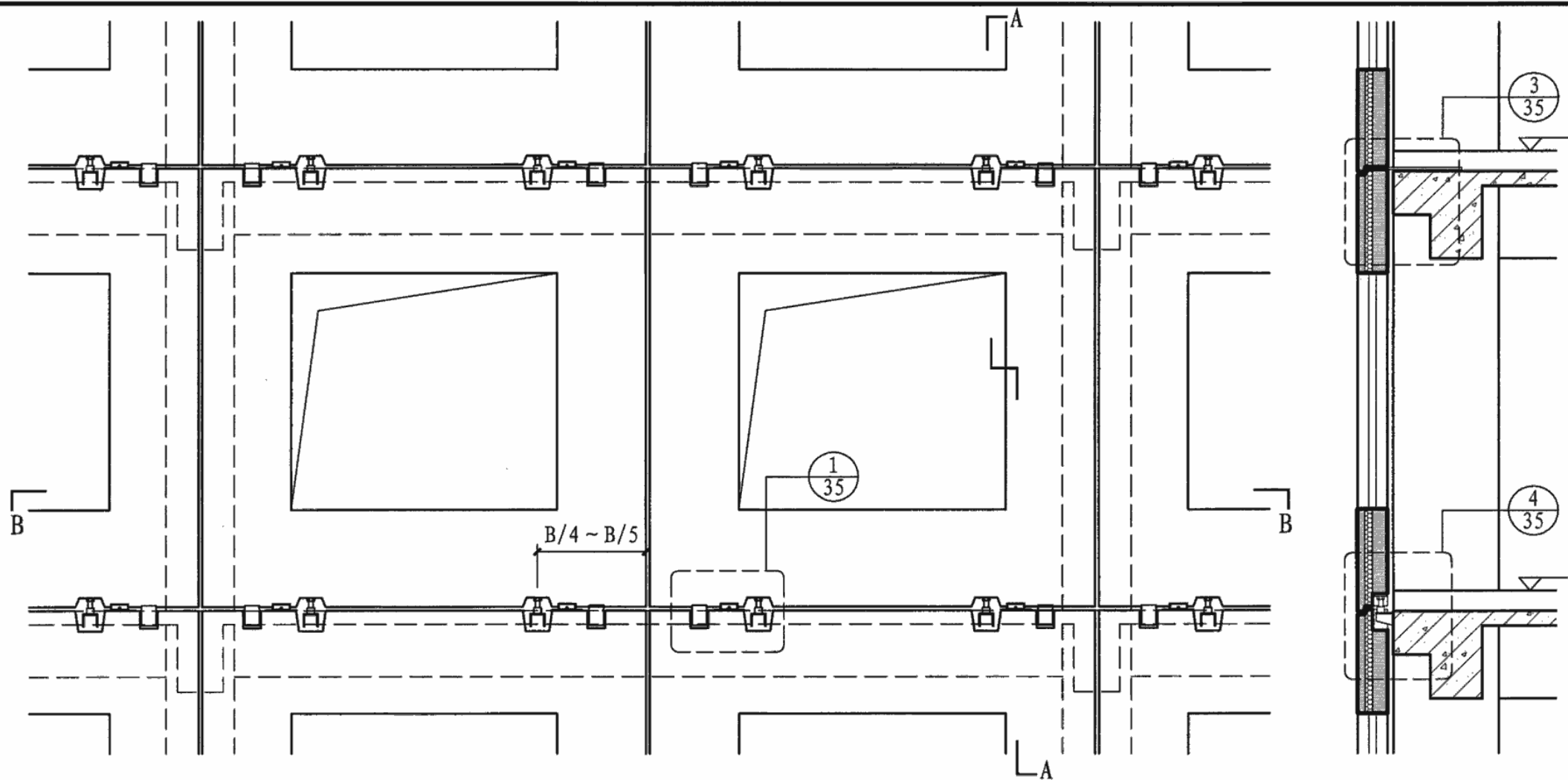
背视图
