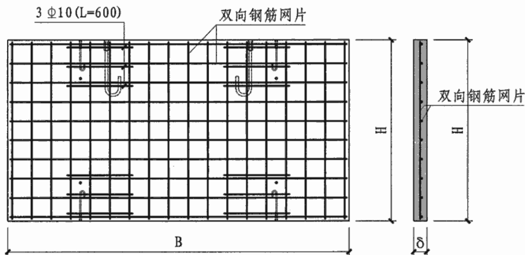
挂板配筋示意
