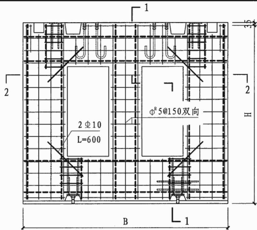
挂板结构层配筋示意
