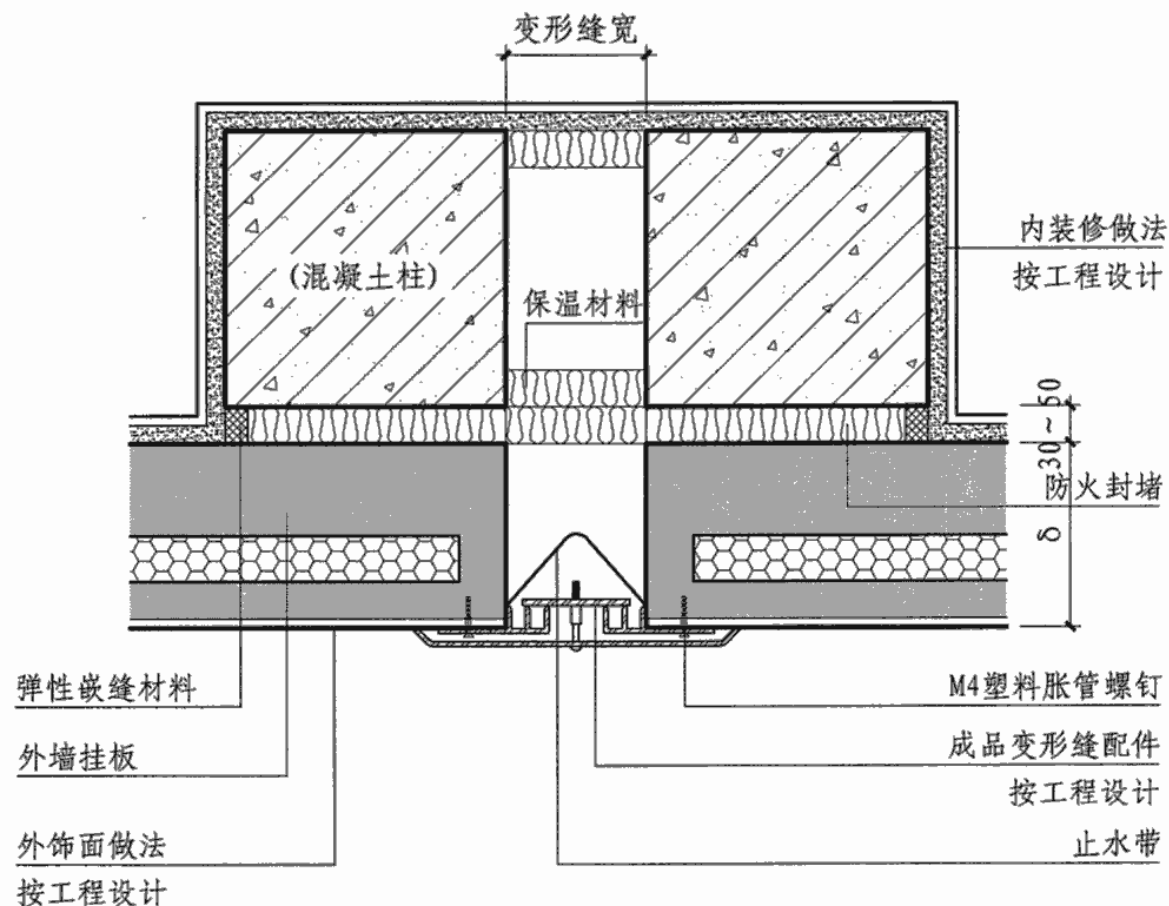
② 变形缝处墙板的构造
