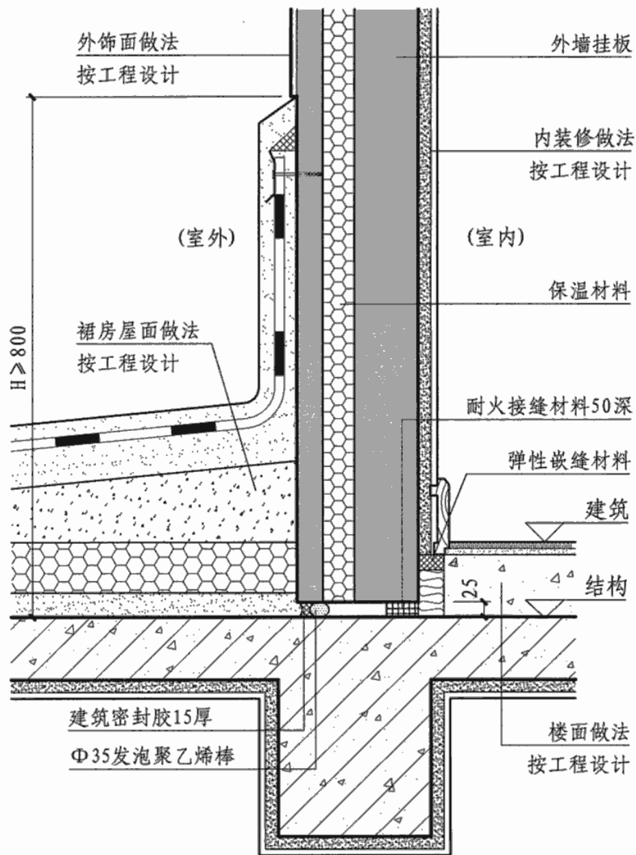
① 裙房屋顶处墙板的构造
