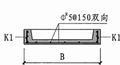
挂板配筋示意
