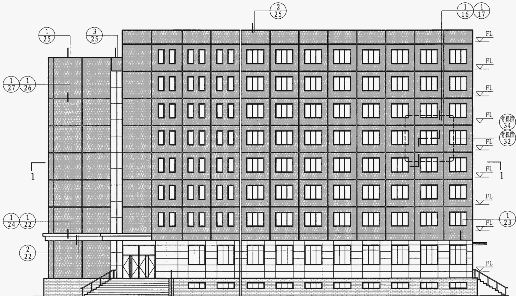
整间板立面
