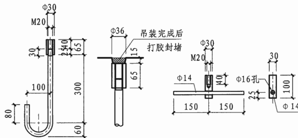
① 安装吊具详图
