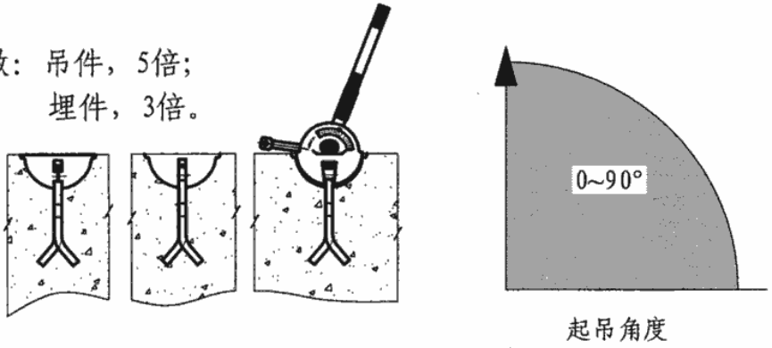
欧瑞提升板件吊具 适合0~90° 起吊
