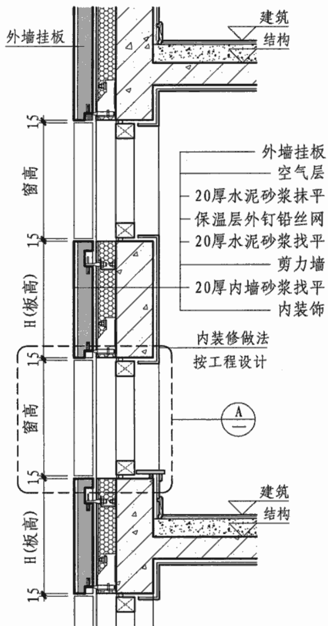
① 装饰板墙身纵剖面
