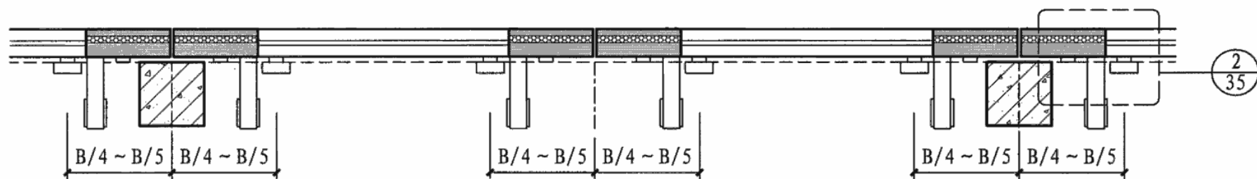
背视图
