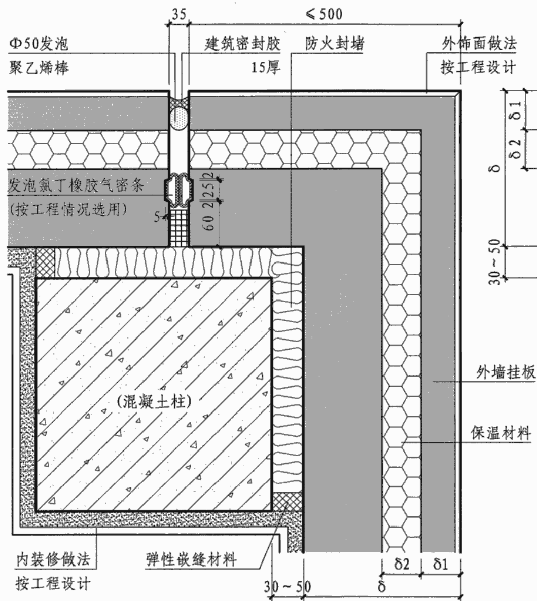
① 外墙挂板阳角横剖面构造
