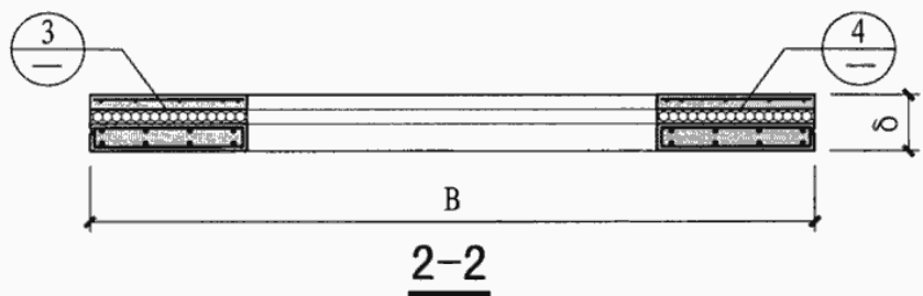
挂板结构层配筋示意
