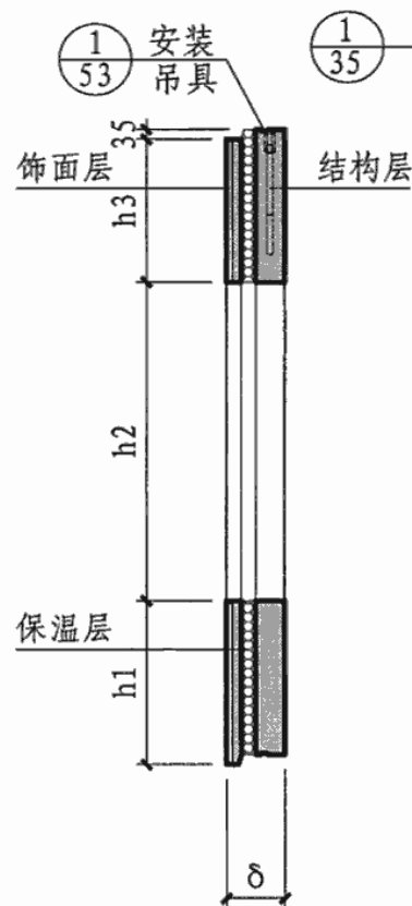
1-1
