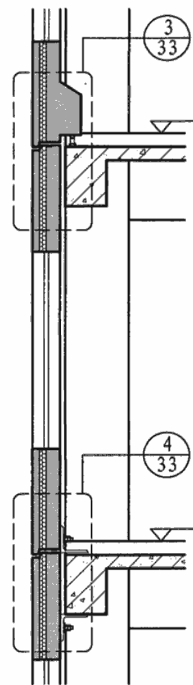
A-A
