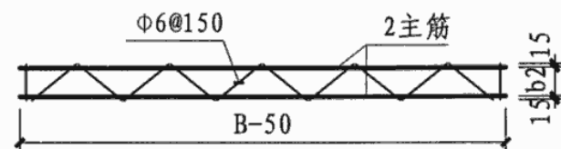
桁架 K2
