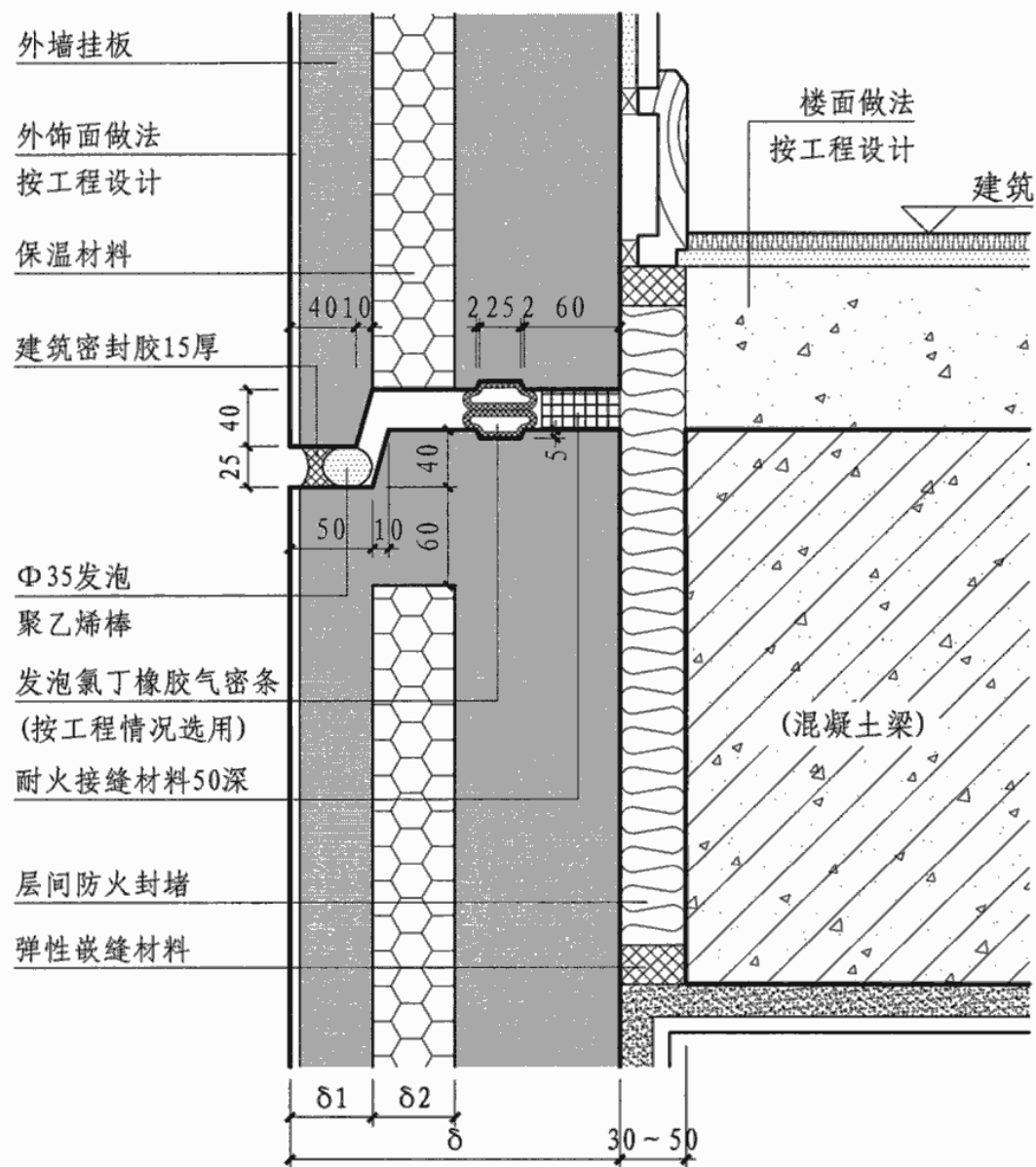
① 外墙挂板水平缝纵剖面构造
