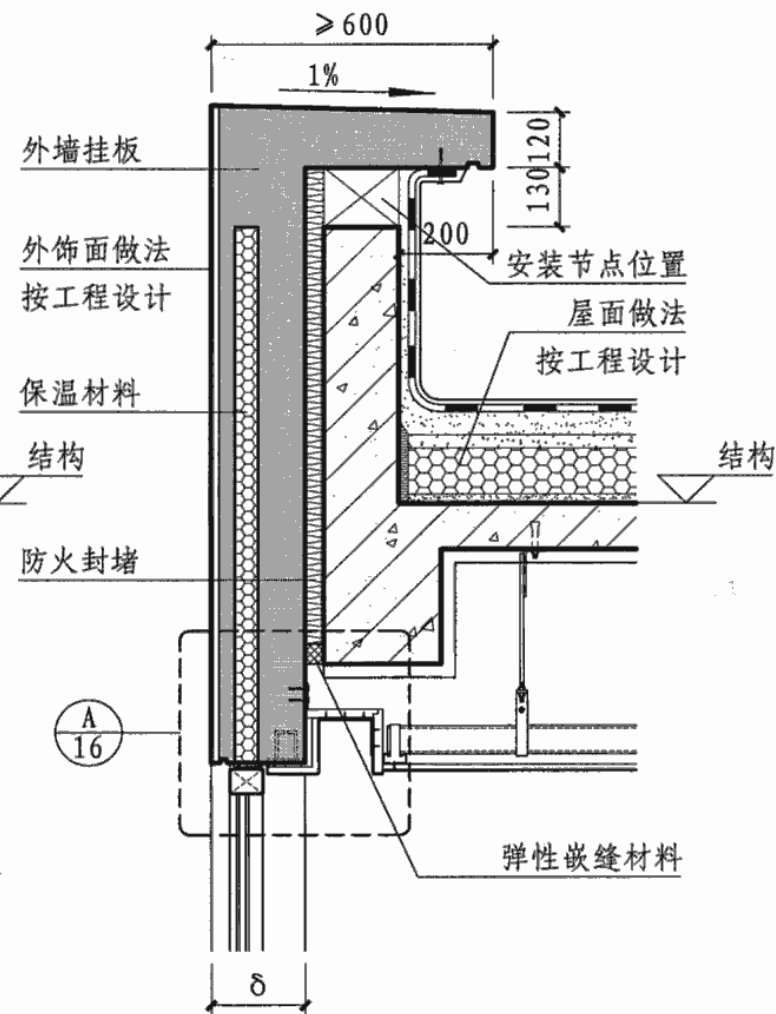
③ 女儿墙墙身剖面详图
