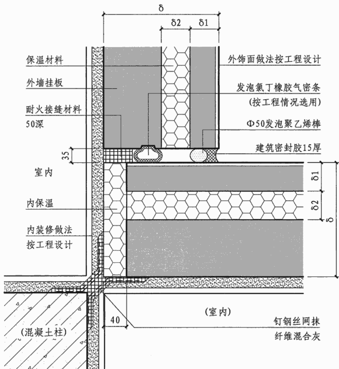
① 外墙挂板阴角横剖面构造
