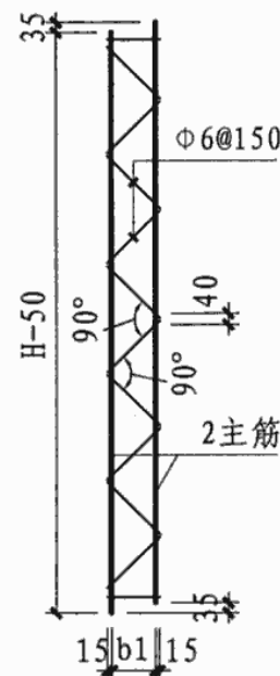
桁架 K1
