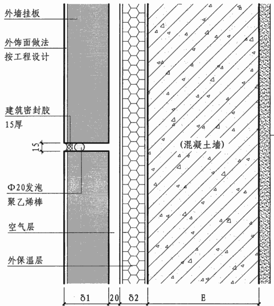
① 外墙挂板水平缝纵剖面构造
